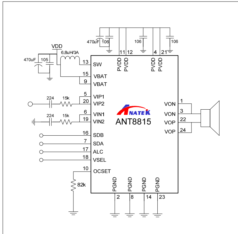
图4. ANT8815 单端输入工作模式电路图
