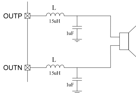
图 7. 负载为 2\Omega \sim 4\Omega 时的 LC 输出滤波器
