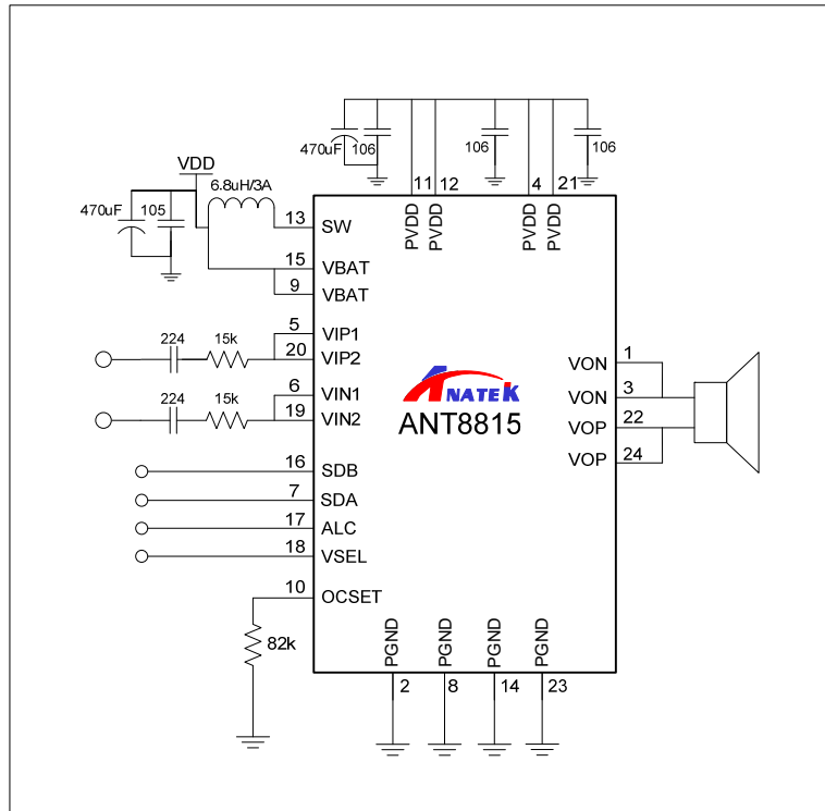
图5. ANT8815 差分输入工作模式电路图
