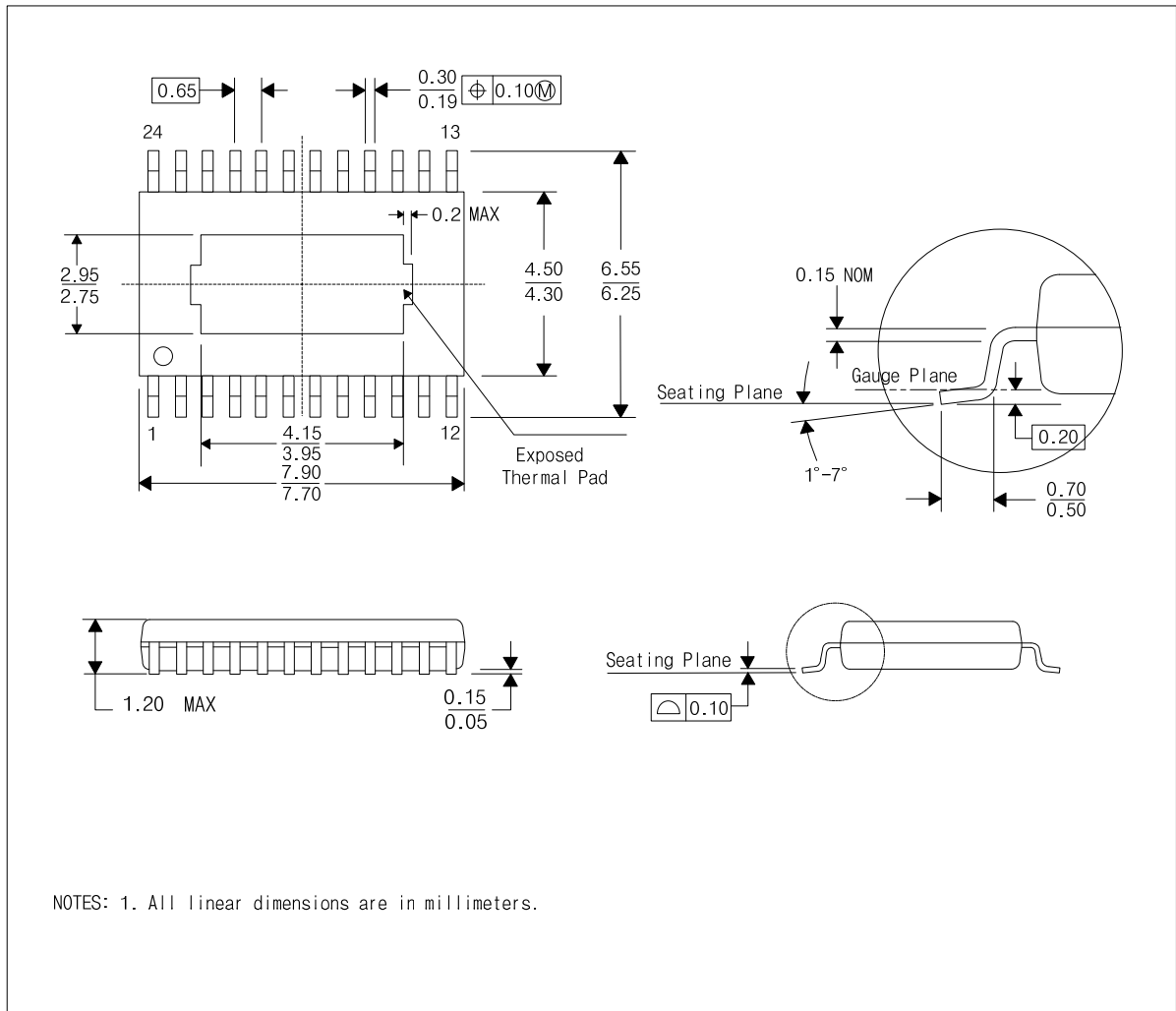
图 8. 封装尺寸图
