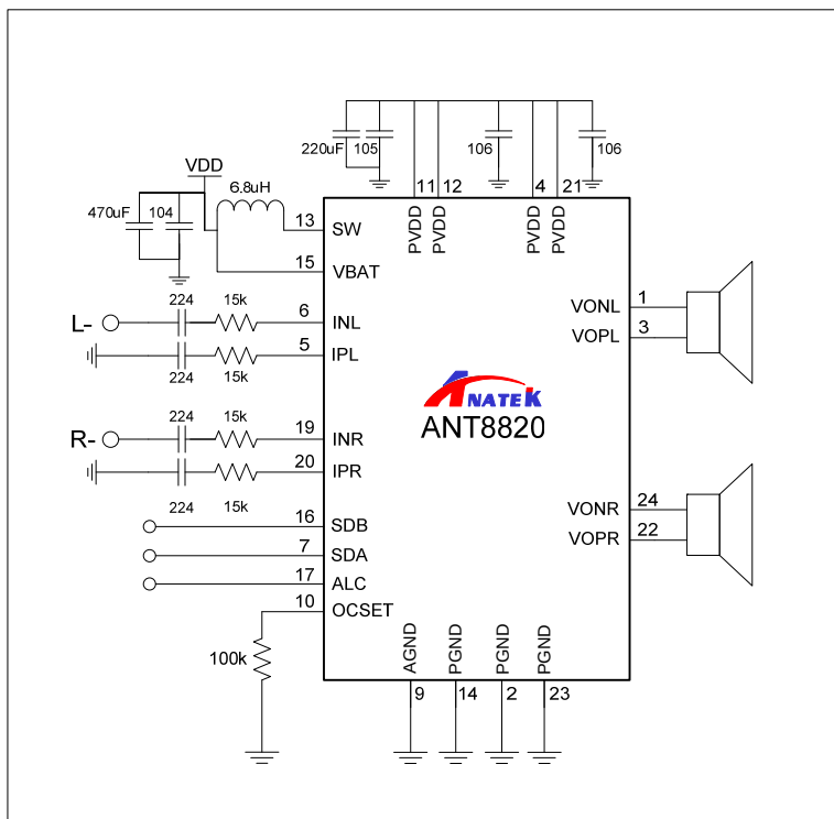
图 4 ANT8820 单端输入工作模式电路图
