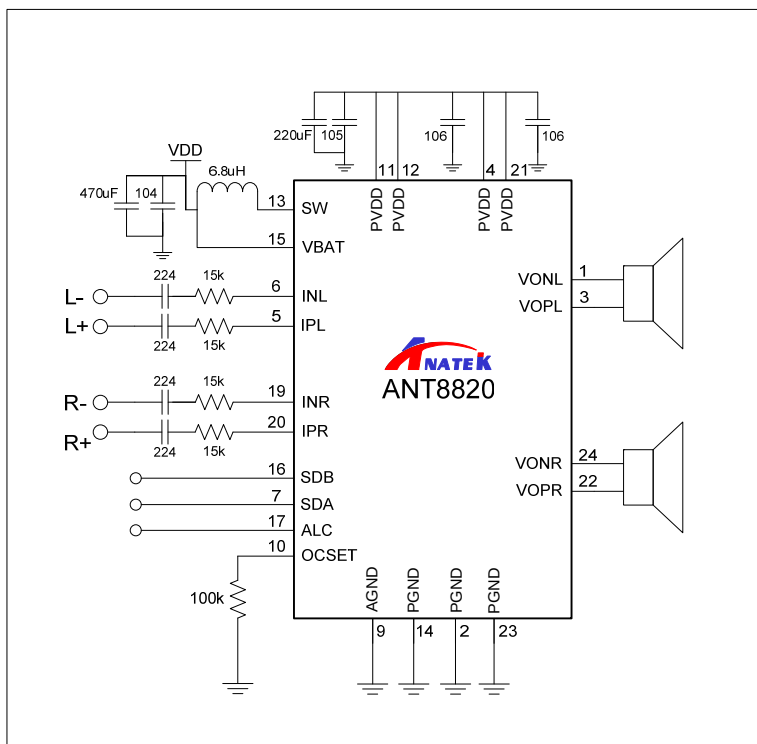
图 5 ANT8820 差分输入工作模式电路图
